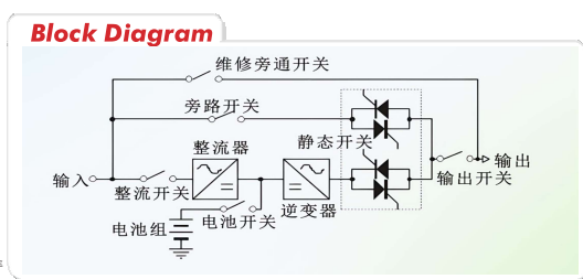
GP 3300 10-40KVA 拓扑图
