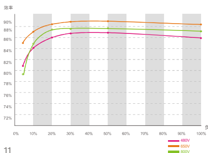
GP 3300 10-40KVA 效率曲线图
